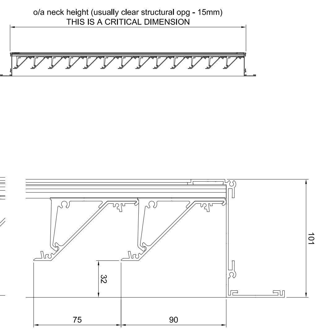
Section A-A ( 1:10 )
